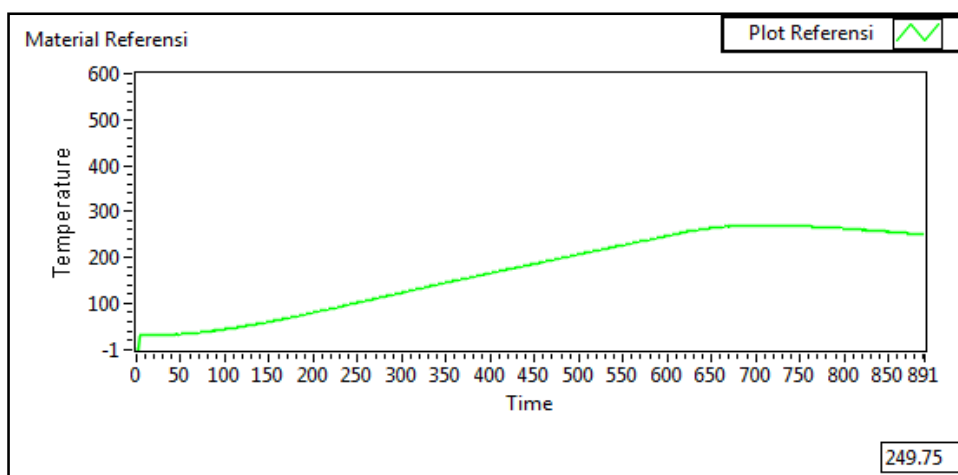
Gambar 12. Grafik Pengujian pada Material Referensi Indium (In)
