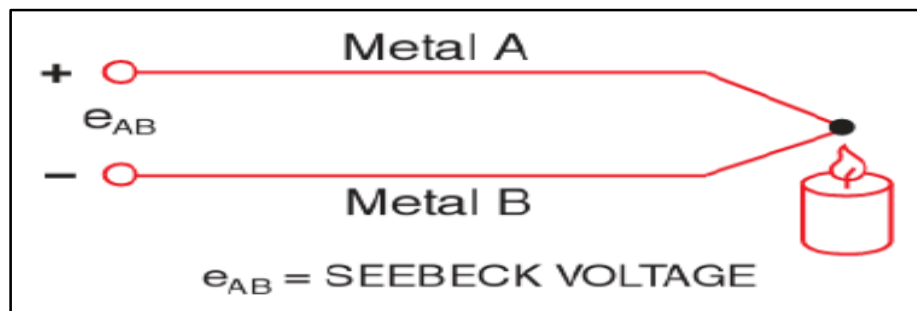
Gambar 2. Tegangan Seebeck yang Muncul Akibat Perubahan Temperatur pada Termokopel
